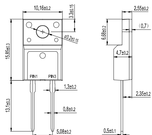
ITO-220AC DR16XXF
